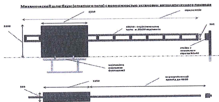
Рис.4. Внешний вид шлагбаума
